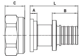
Перехідник із накидною гайкою під плоске ущільнення КА.А08F-16S – КА.А08F-25S
